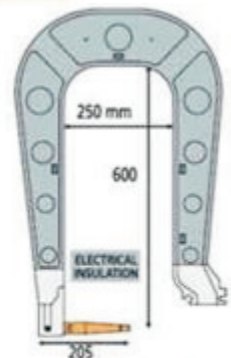
C9 Ref 020078 8 bar / 550 daN
